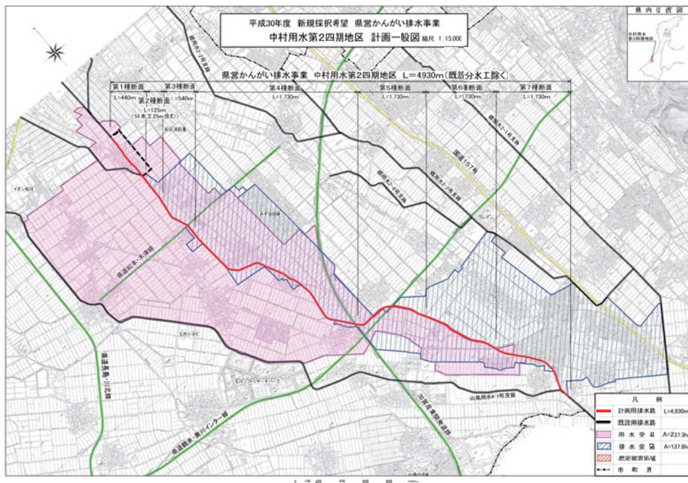
中村用水第2四期地区 計画一般図
